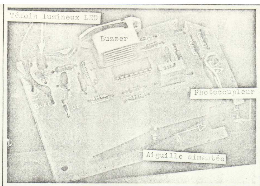
L'ensemble monté (hors coffret)
